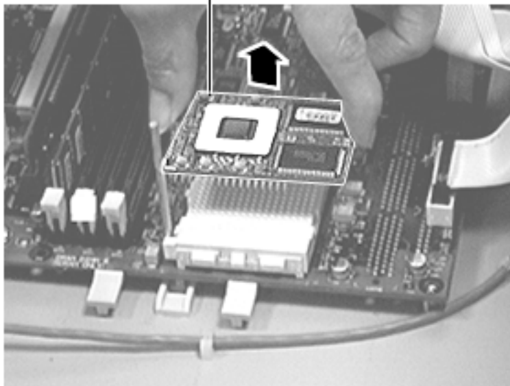
Processor Module
