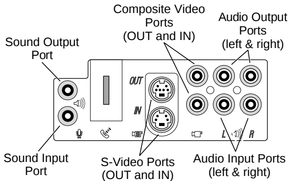
AV I/O Panel (Power Macintosh G3 Minitower Only)
