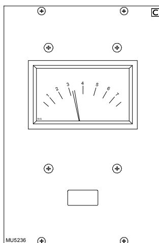
PPM Meter
