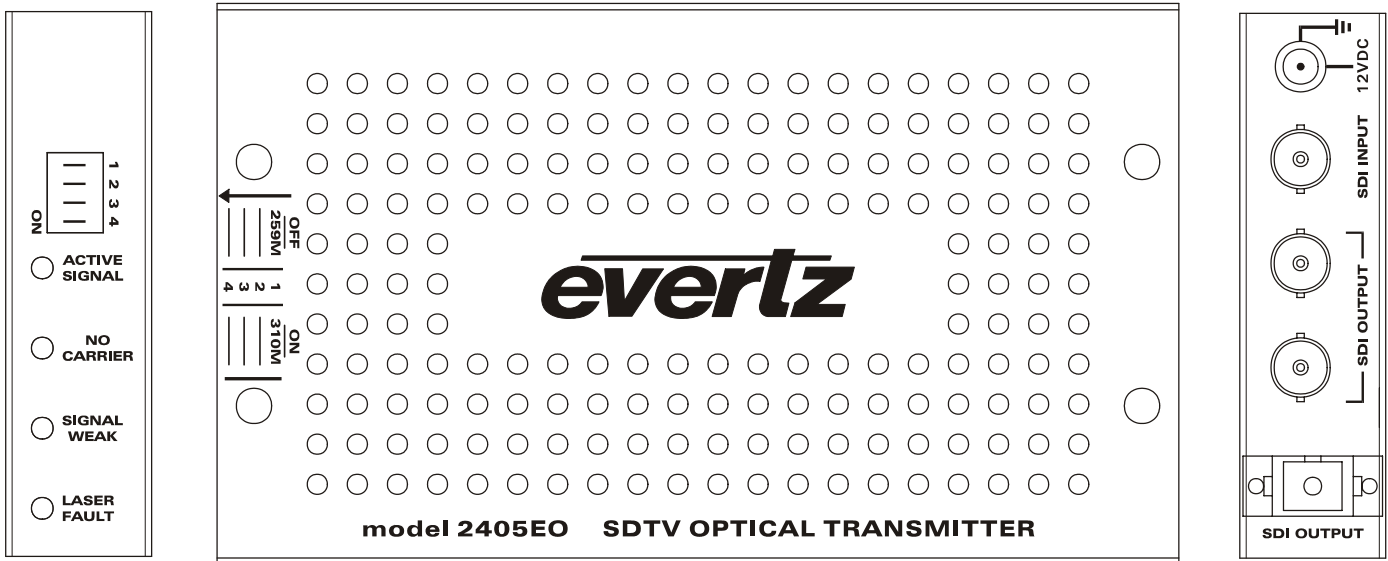
Figure 2-1: 2405EO Module
