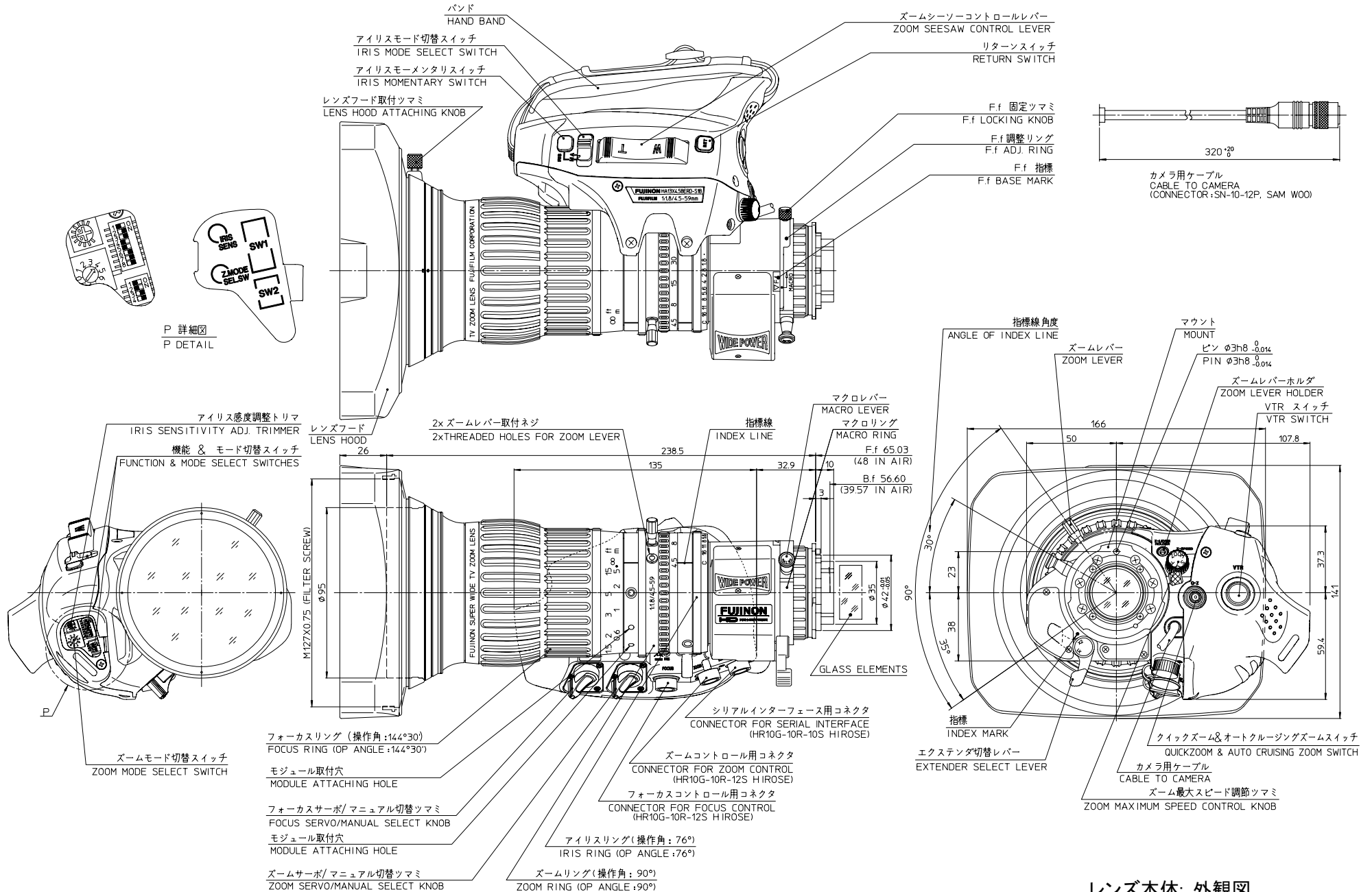
レンズ本体: 外観図 Outline drawing HA13×4.5BERD-S1B
