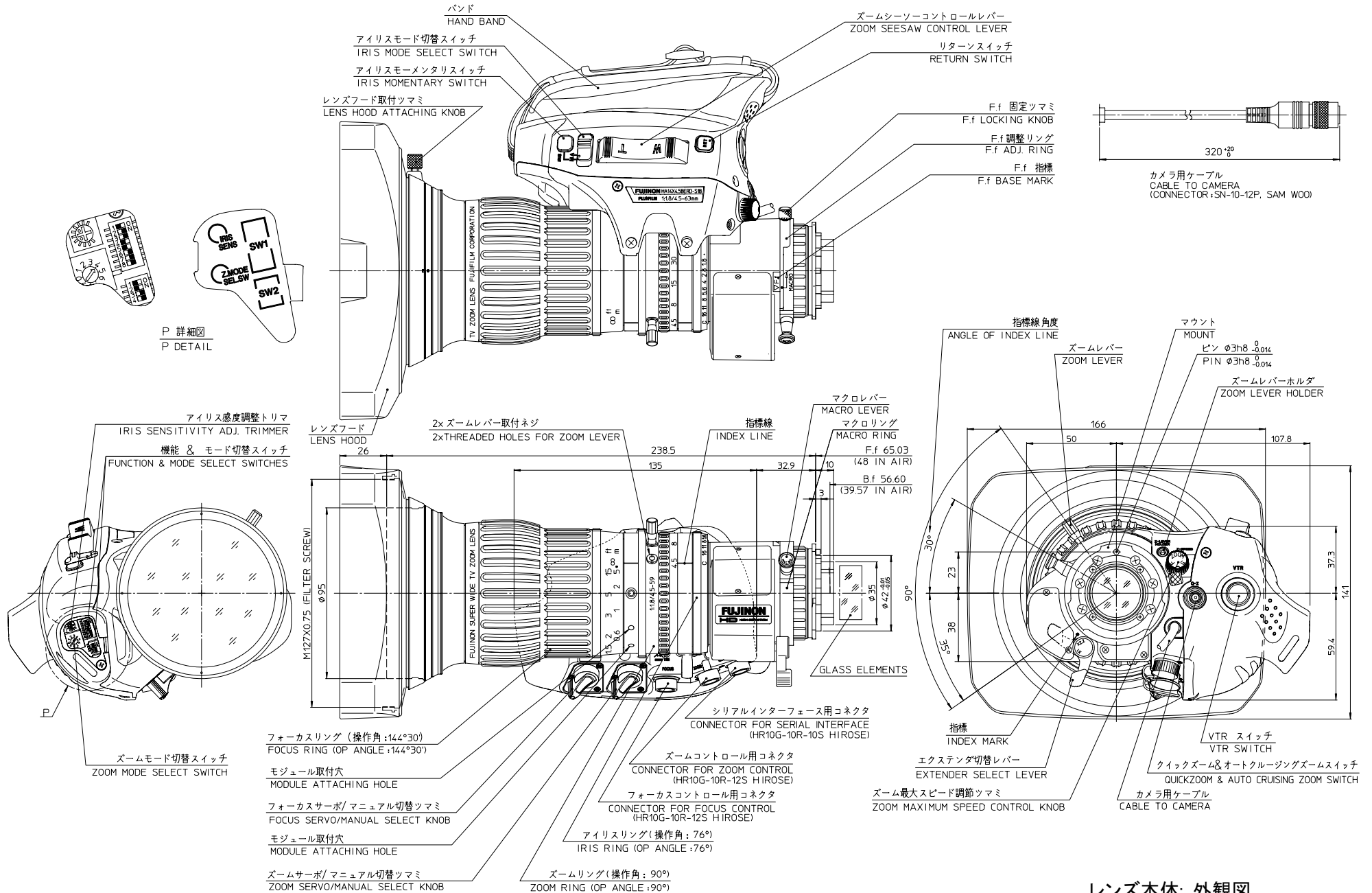
レンズ本体: 外観図 Outline drawing HA14×4.5BERD-S1B
