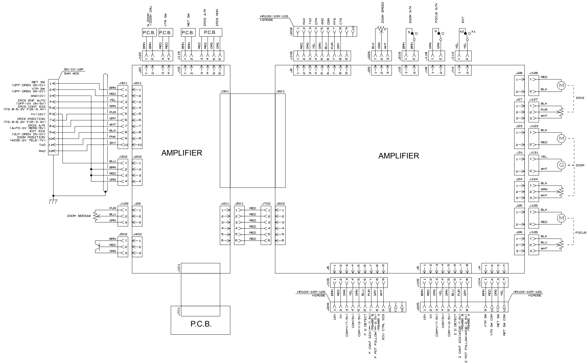
ドライブユニット: 結線図 Drive unit: wiring diagram
