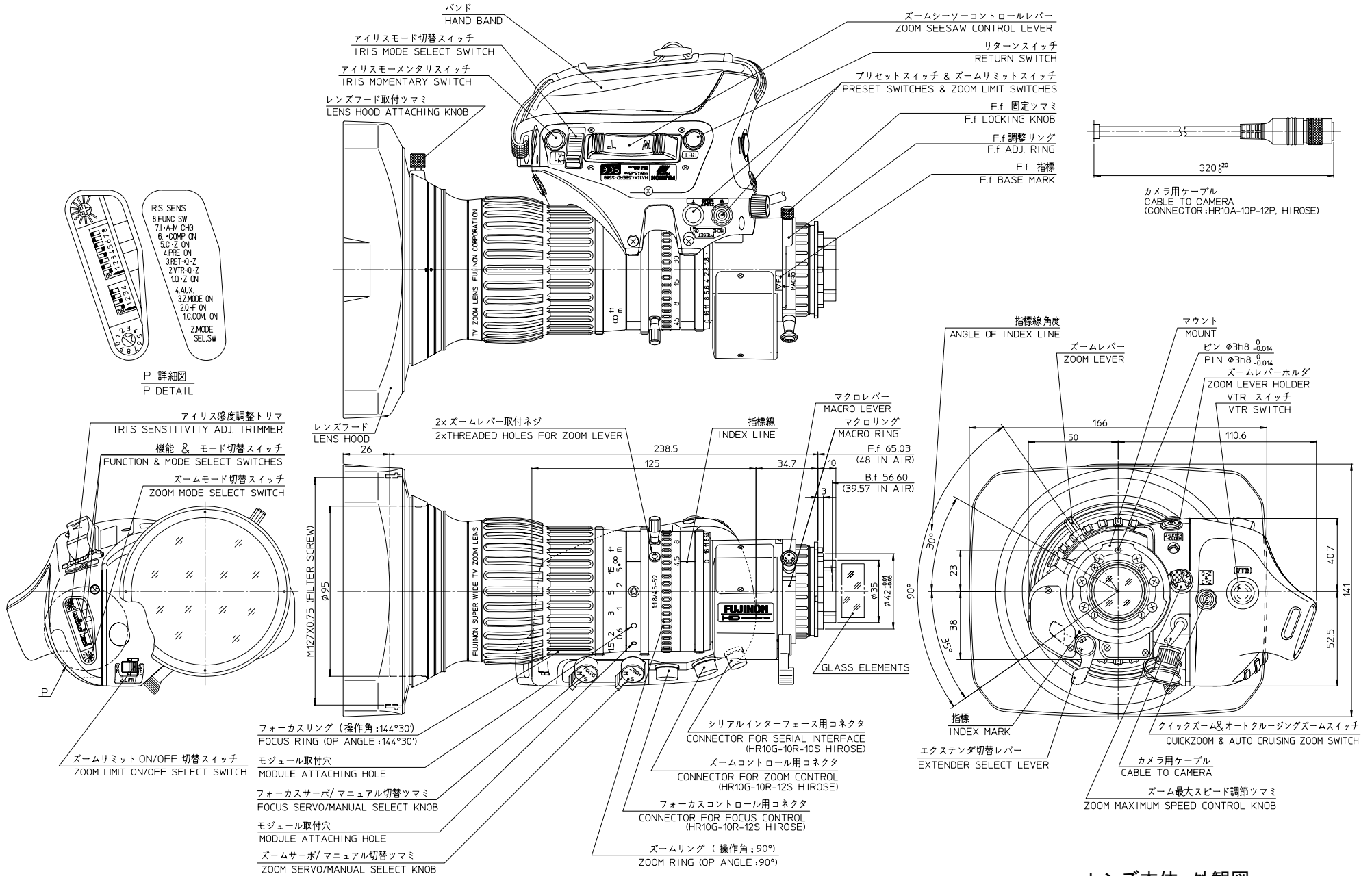
レンズ本体: 外観図 Outline drawing HA14×4.5BERD-S58B
