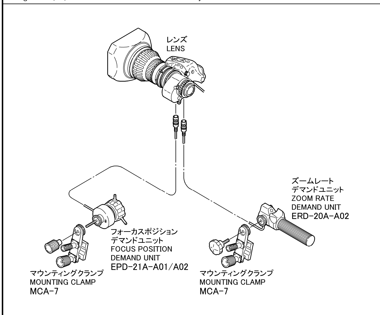
システム図 (例) Configuration (Ex.)
