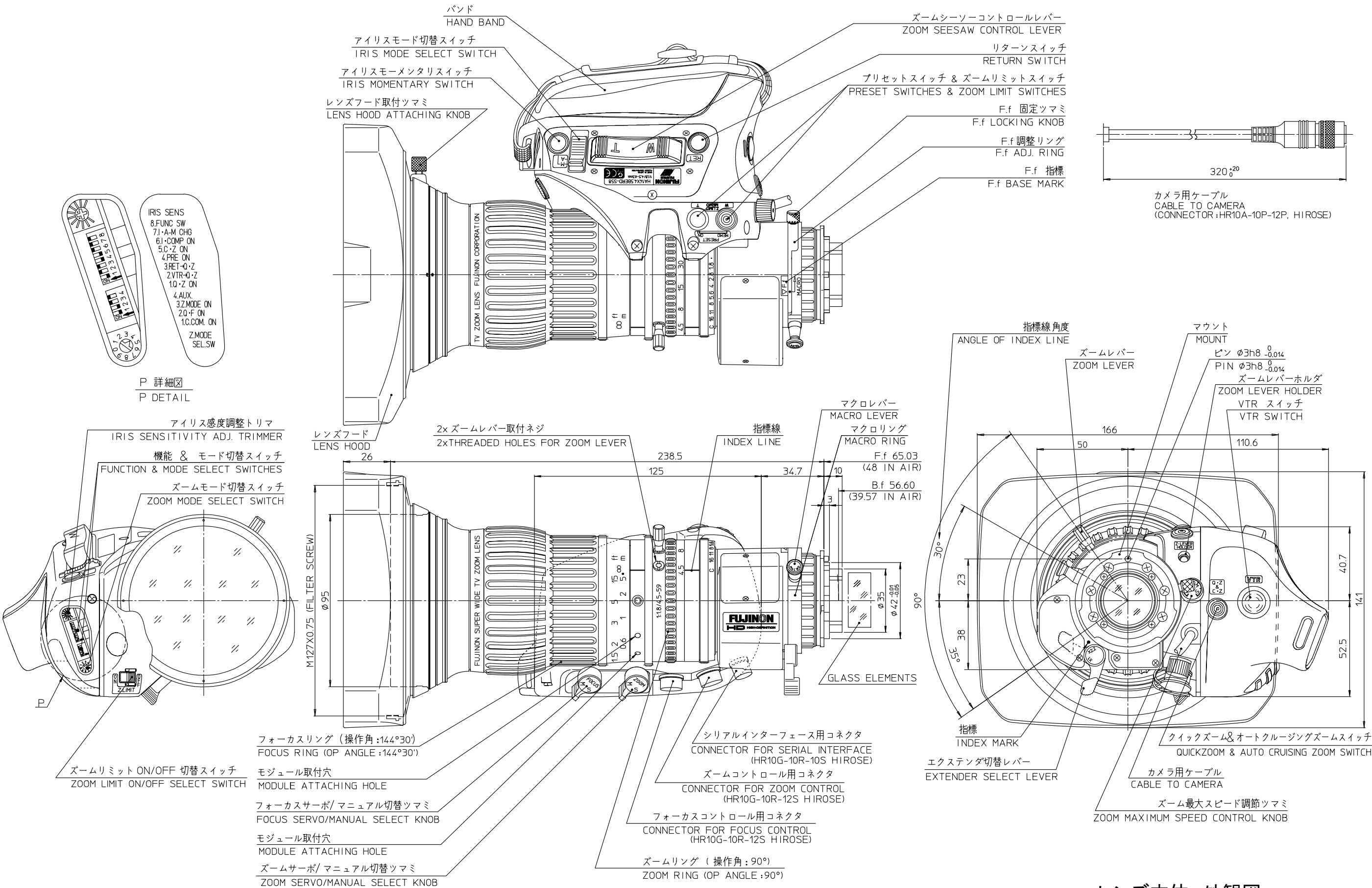
レンズ本体: 外観図 Outline drawing HA14×4.5BERD-S58
