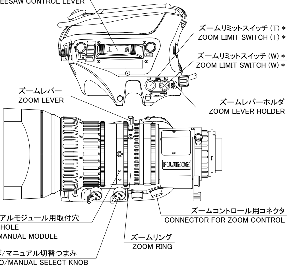
ズームシーソーコントロールレバー ZOOM SEESAW CONTROL LEVER
