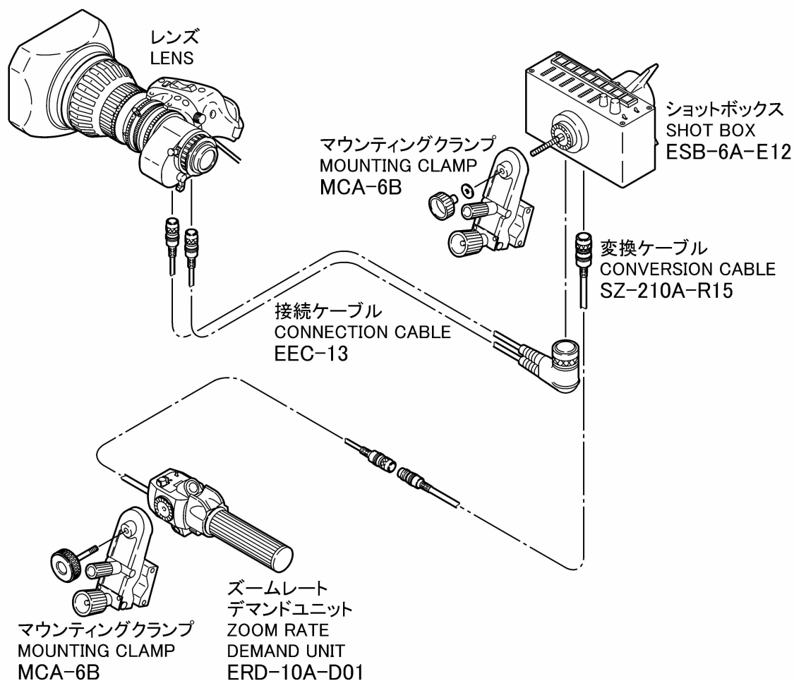
システム図 Configuration
