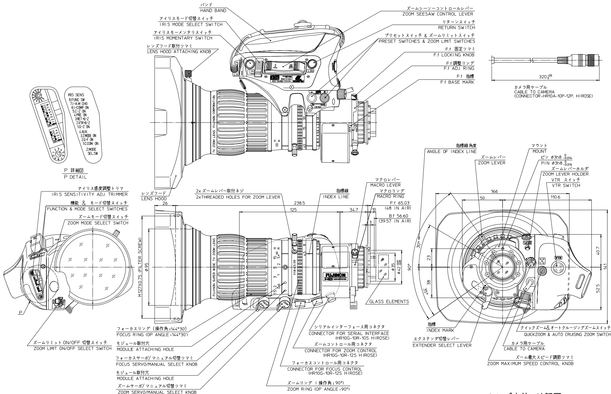
レンズ本体: 外観図 Outline drawing HA14×4.5BERD-S58
