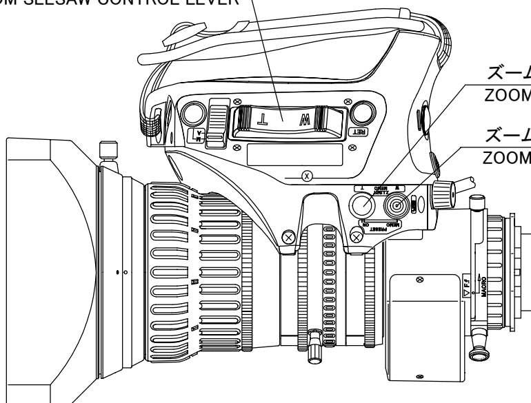
ズームシーソーコントロールレバー ZOOM SEESAW CONTROL LEVER
