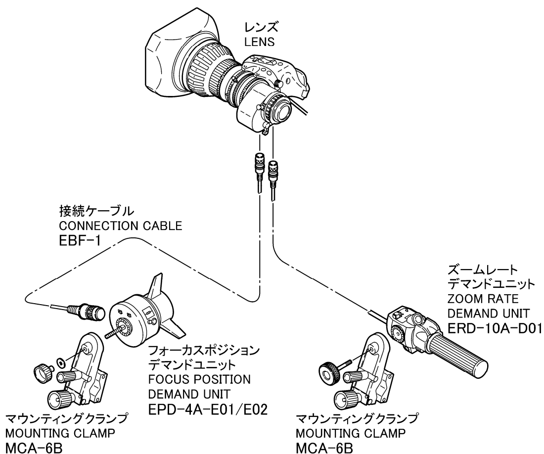
システム図 Configuration
