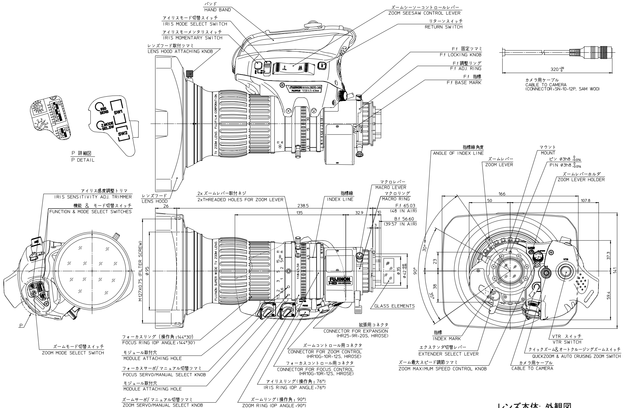
レンズ本体: 外観図 Outline drawing HA14×4.5BERD-S6B
