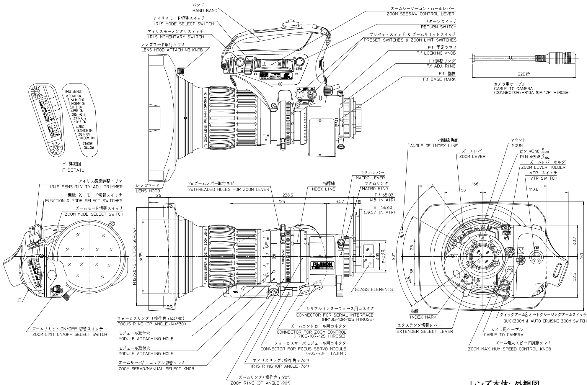
レンズ本体: 外観図 Outline drawing HA14×4.5BERM-M58B
