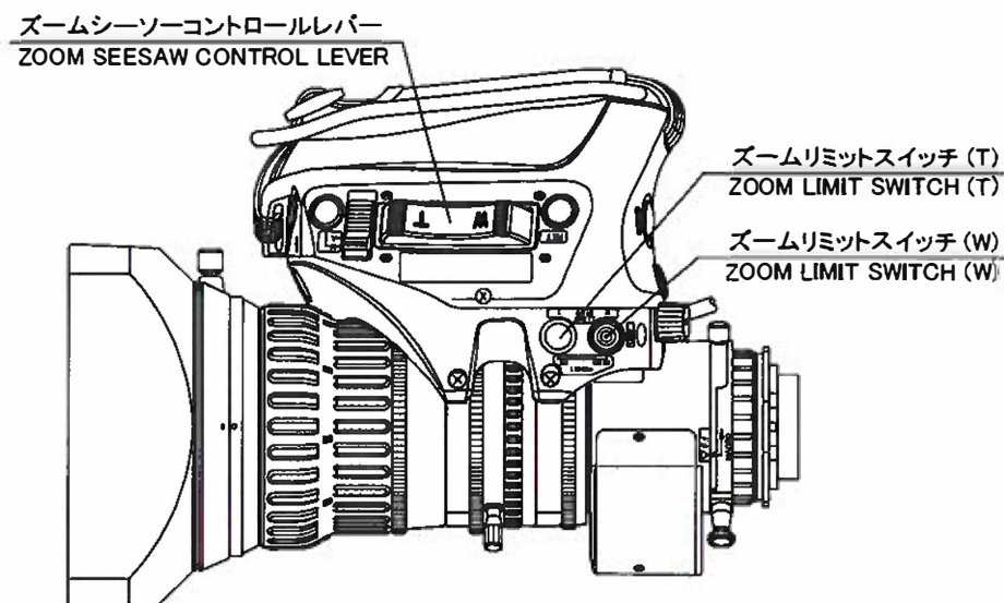
上面図/Top View
