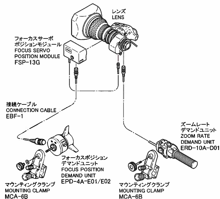
システム図 Configuration
