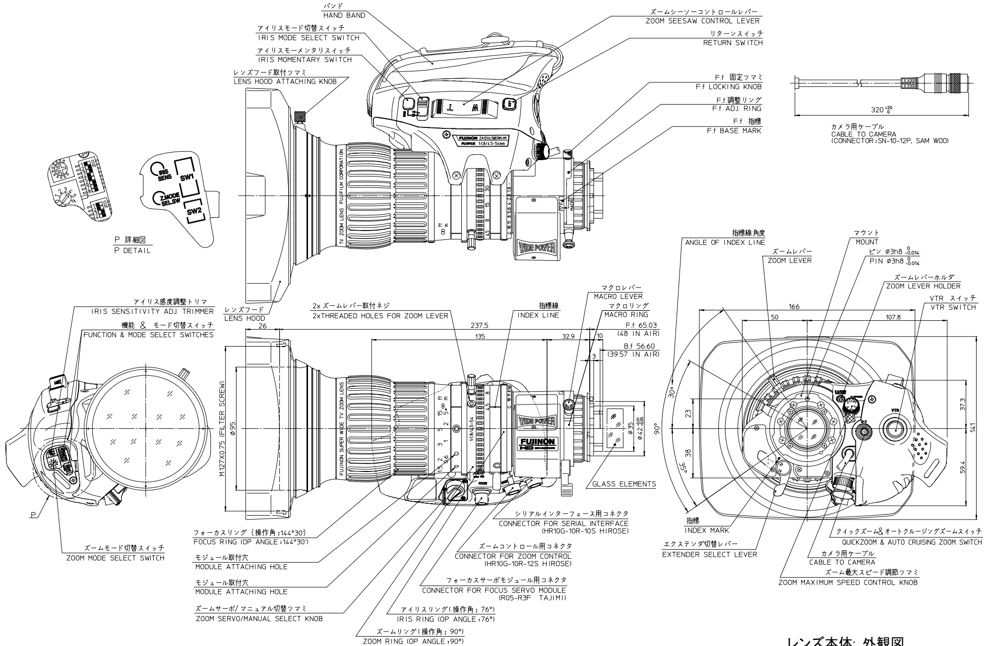
レンズ本体: 外観図 Outline drawing ZA12×4.5BERM-M1
