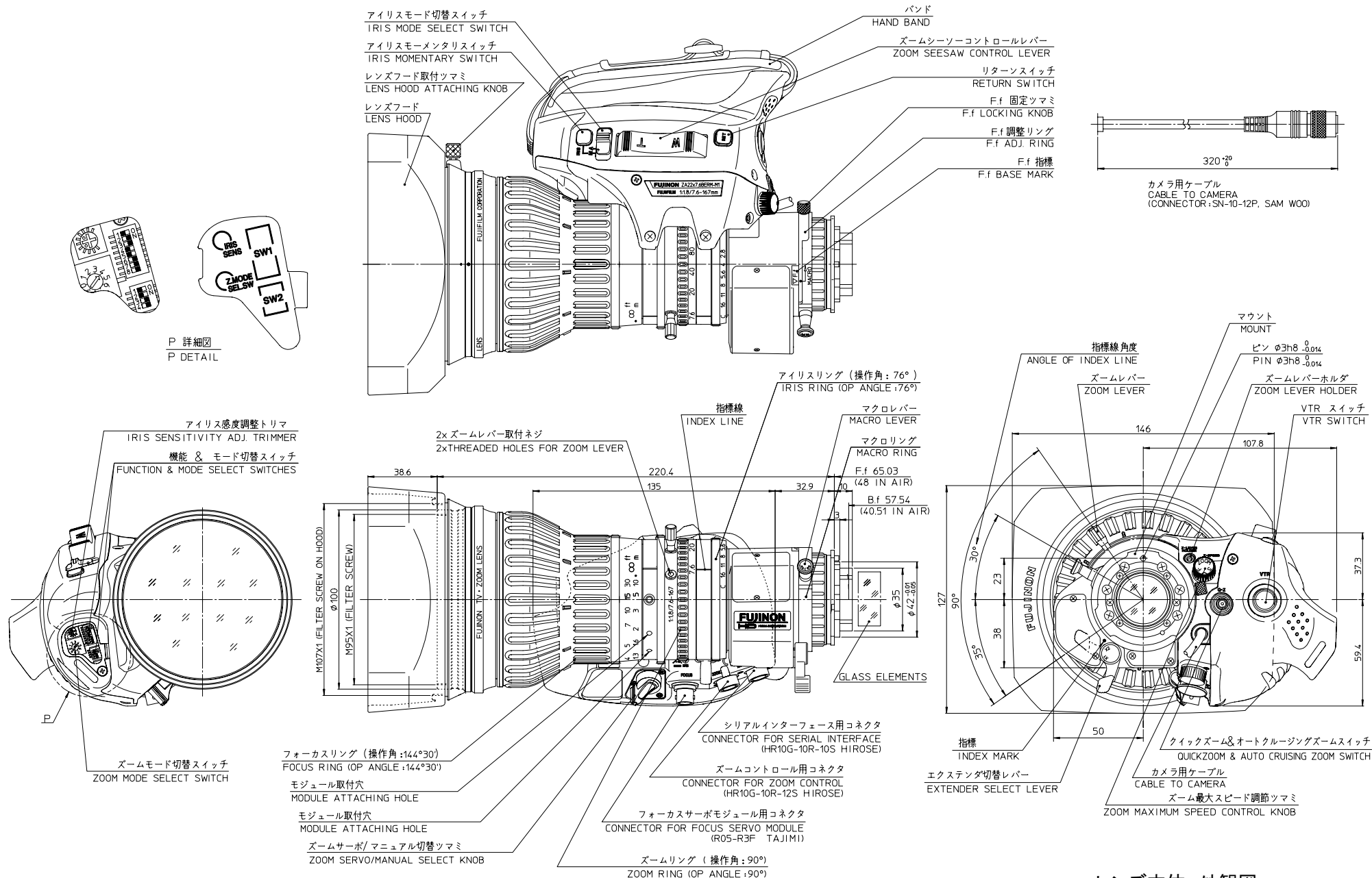
レンズ本体: 外観図 Outline drawing ZA22×7.6BERM-M1
