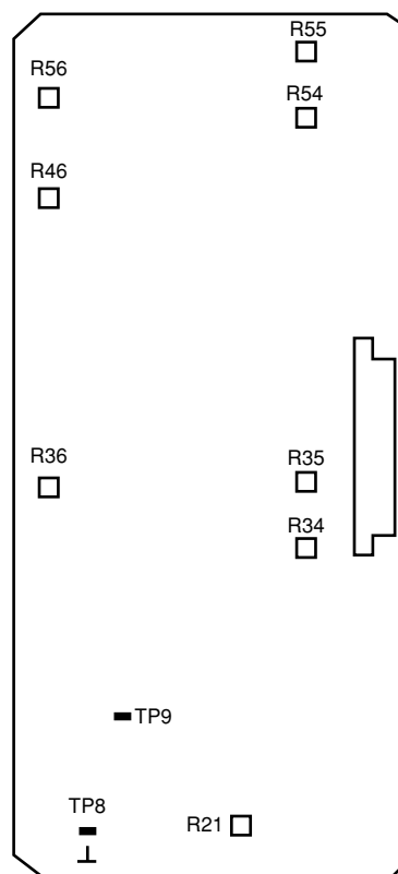
«AP1 PCB»
