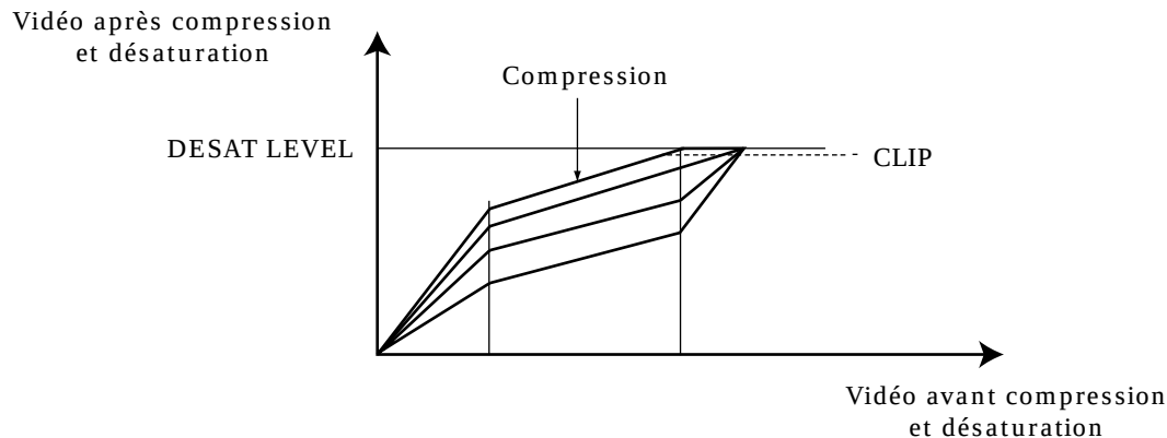
RÉPONSE DES ÉTAGES DE COMPRESSION ET DÉSATURATION
