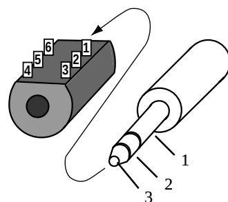
Embase type "JACK" Prise correspondante: -Type: JACKFLJCN -Réf: T1004861
