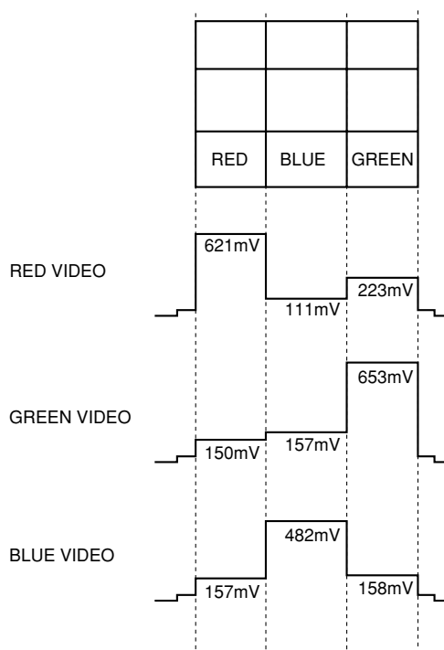
Niveaux théoriques de réglage du MASKING
