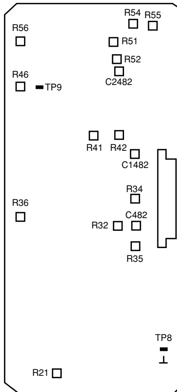
«AP PCB»
