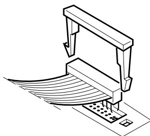
- J03 «SUPÉRIEUR» PCB
