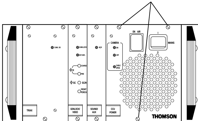
Vis de fixation de l'ensemble CCU POWER
