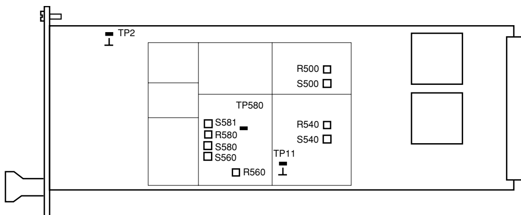
«SOUND / AUX PCB»
