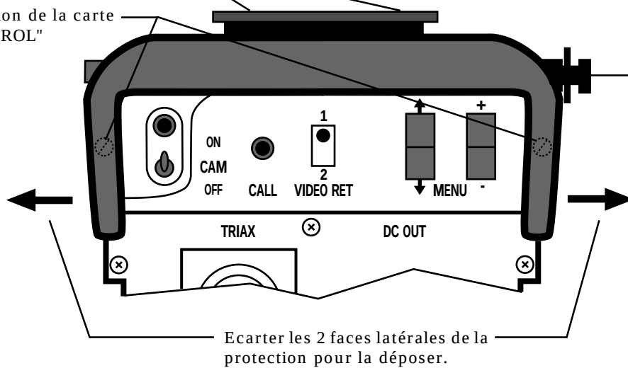
DÉPOSE DE LA CARTE "REAR CONTROL"
