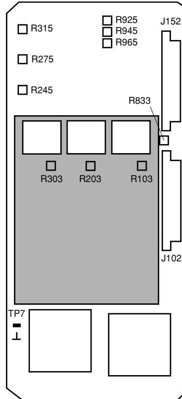
«DP1 PCB»
