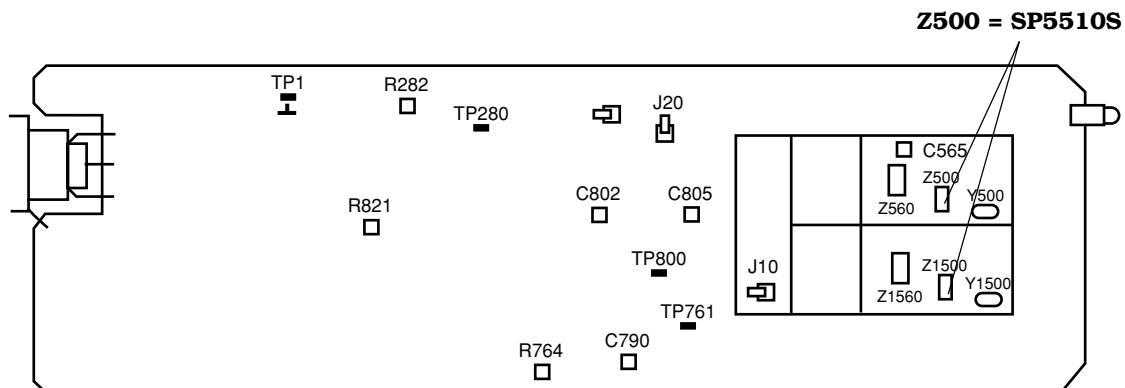
«TRIAX PCB» VERSION 1
