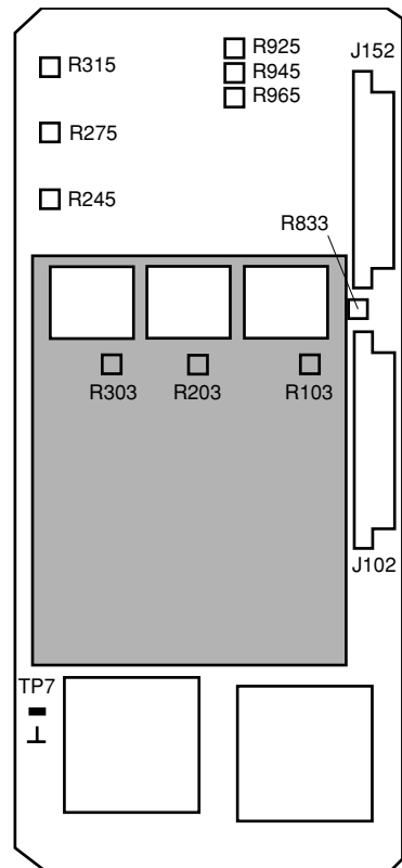
«DP1 PCB»
