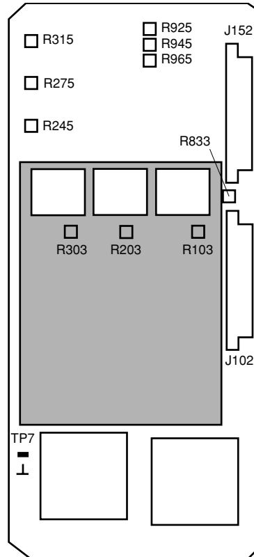
«DP1 PCB»
