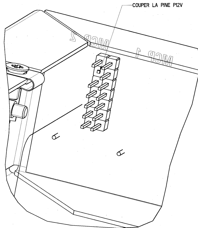
DETAIL A VUE DE L'INTERIEUR DU CAISSON CARTE CONNECTION ADAPTATOR PANEL
