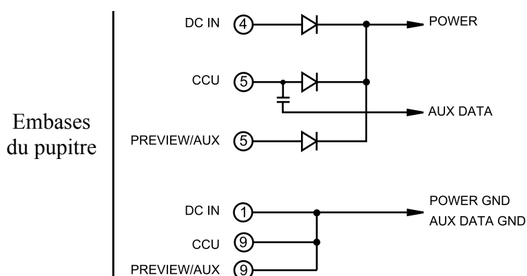
Figure 1 : Connection des différentes alimentations du pupitre
