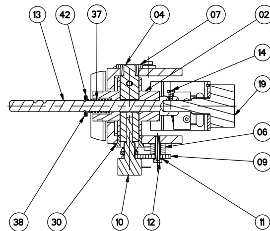
COUPE B-B
