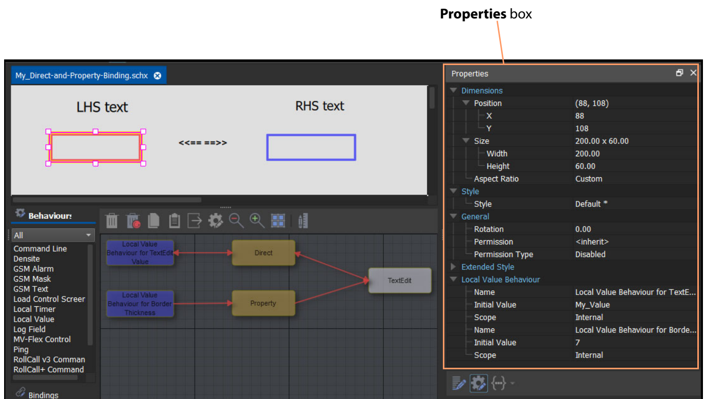
Fig. 3-1: Properties Box
