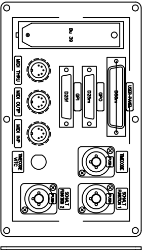
Schematische Ansicht
