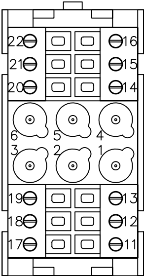
HARTING SCHRAUBANSCHLUSS K6/12 432.4170
