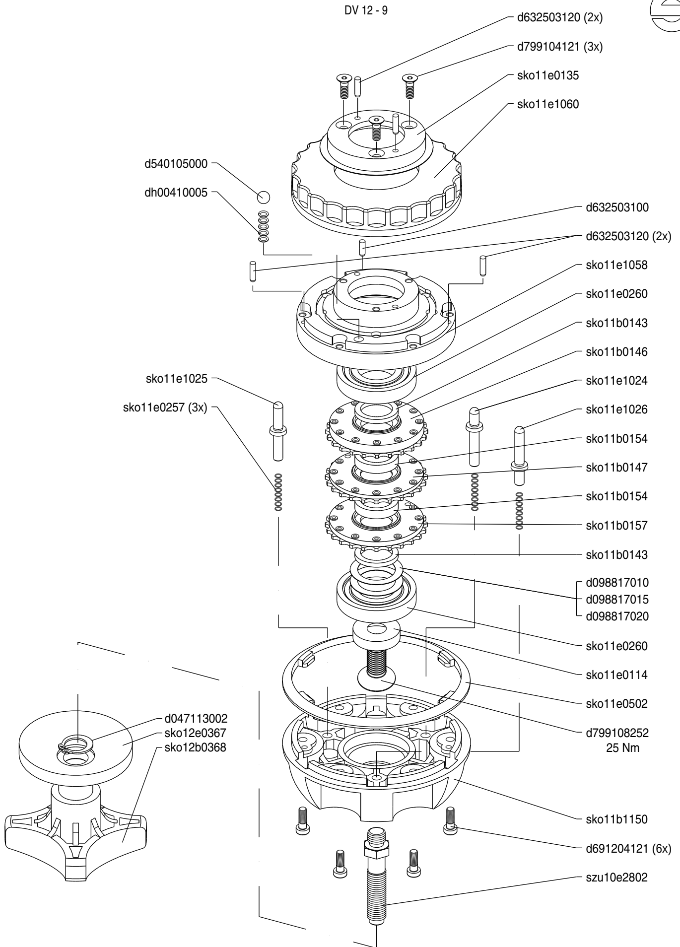
Halbkugel mit Dämpfungspaketen Ball assembly with fluid modules
