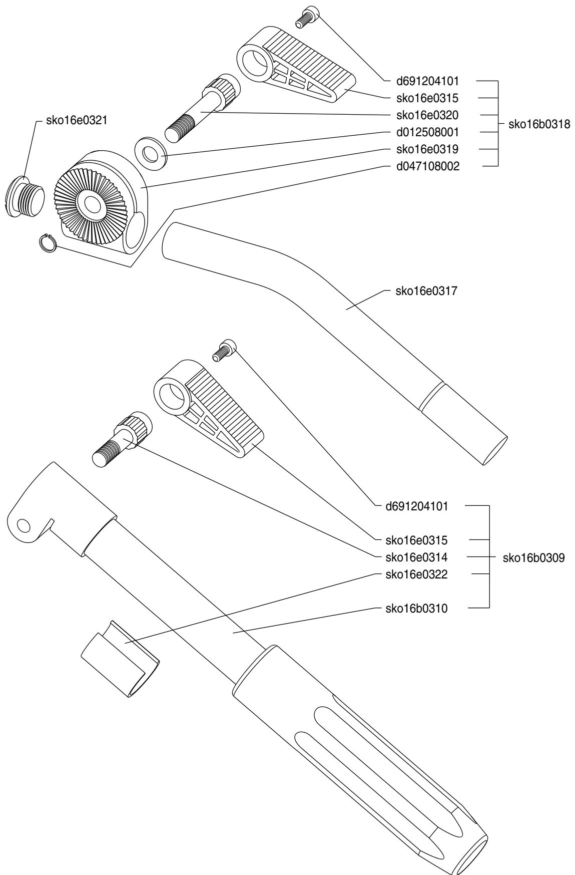
Schwenkarm rechts 3070 Pan bar right 3070
