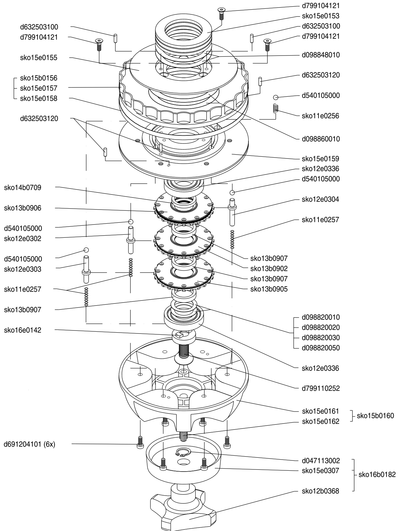
Halbkugel mit Dämpfungspaketen Ball assembly with fluid modules
