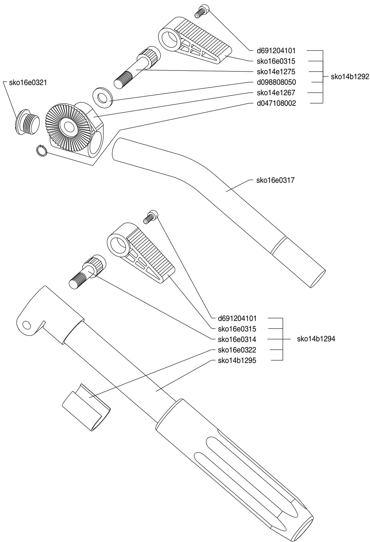
Schwenkarm Plus rechts Pan bar plus right
