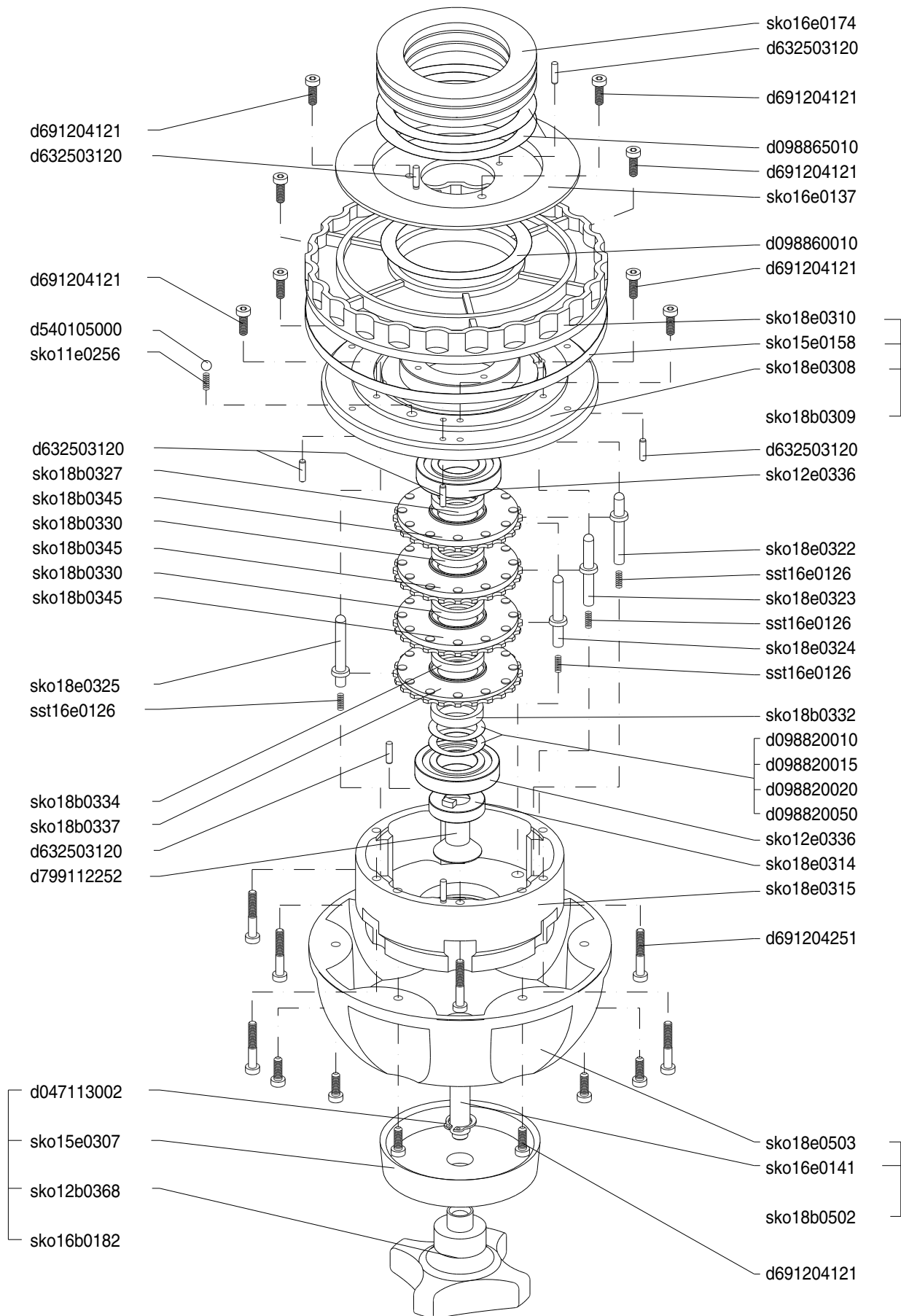
Halbkugel mit Dämpfungspaketen 150mm Ball assembly with fluid modules
