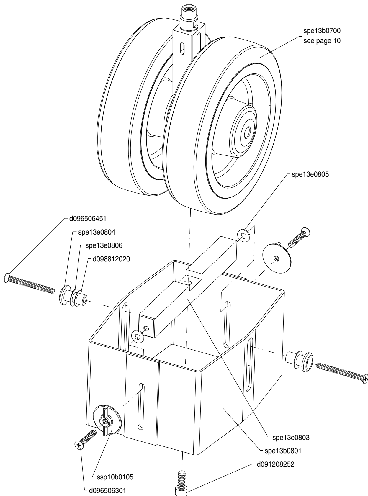
Laufrolle Ö200 mit Kabelschutz spe13b0800 Wheel assembly Ö200 with cable guard
