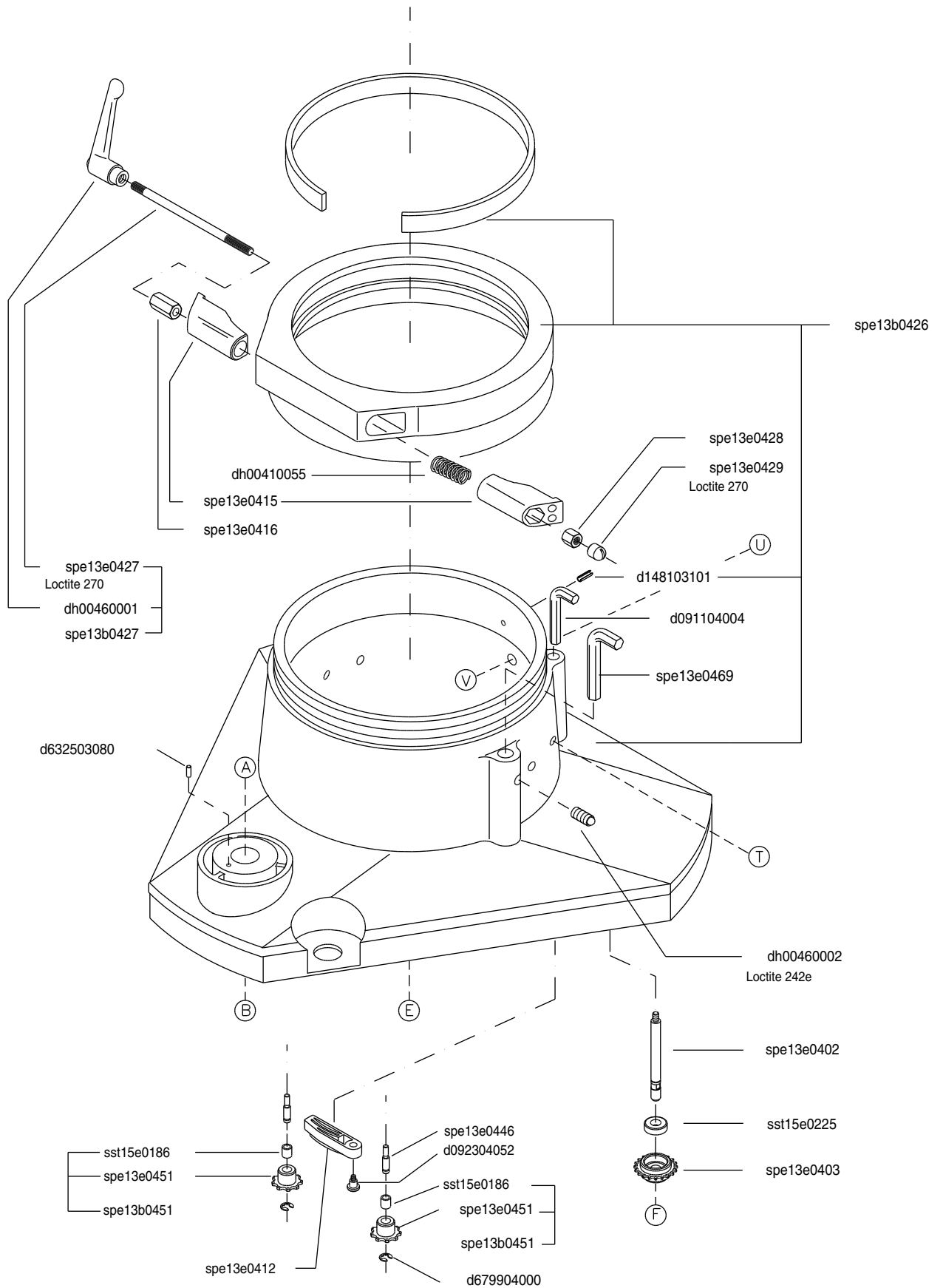
Vario - Pedestal Flansch mit Klemmring flange with lock collar
