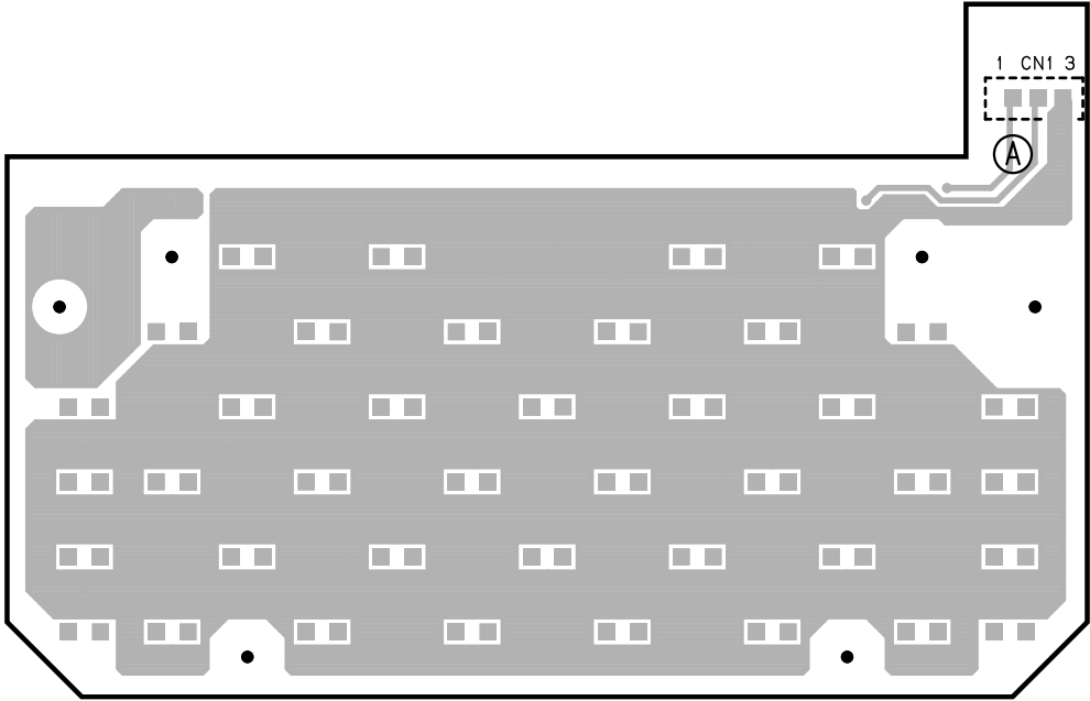
LE-172 -A SIDE- SUFFIX : -13 LE-216 -A SIDE- SUFFIX : -11
