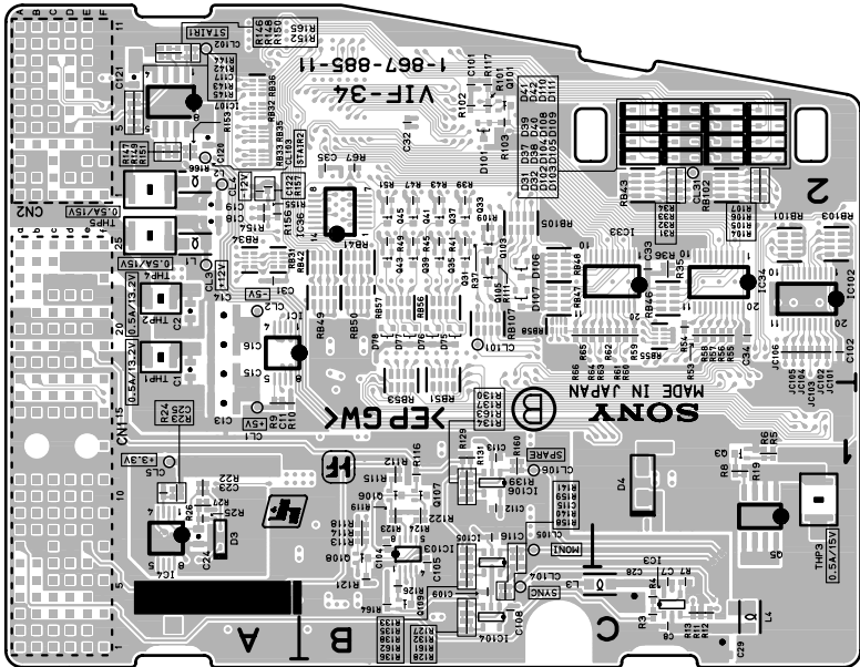
VIF-34 VIF-34B -B SIDE- SUFFIX: -11, 31
