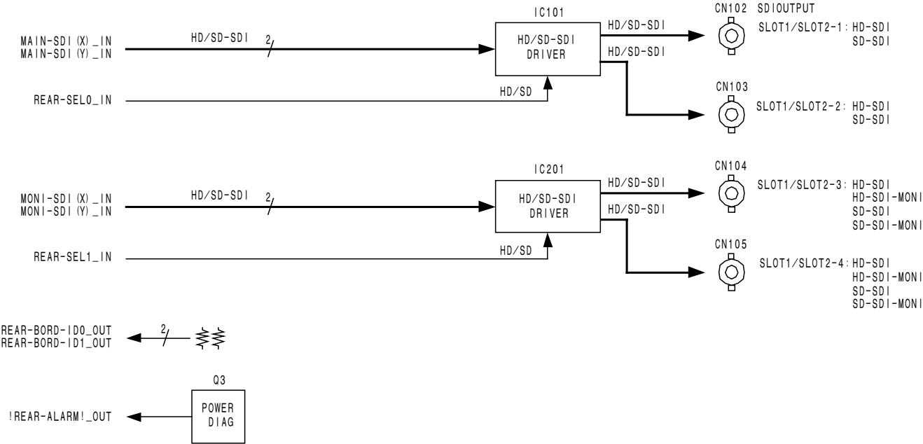
SDI OUTPUT HIF-25
