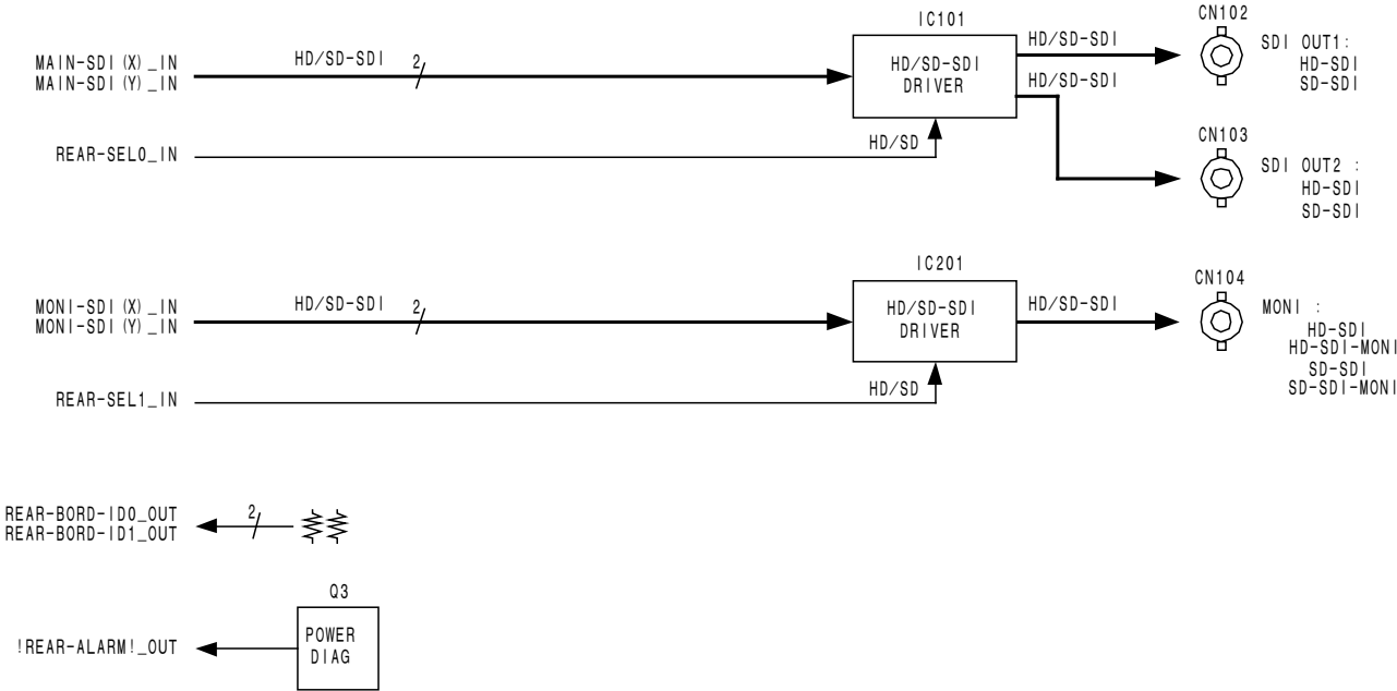
SDI OUTPUT HIF-27
