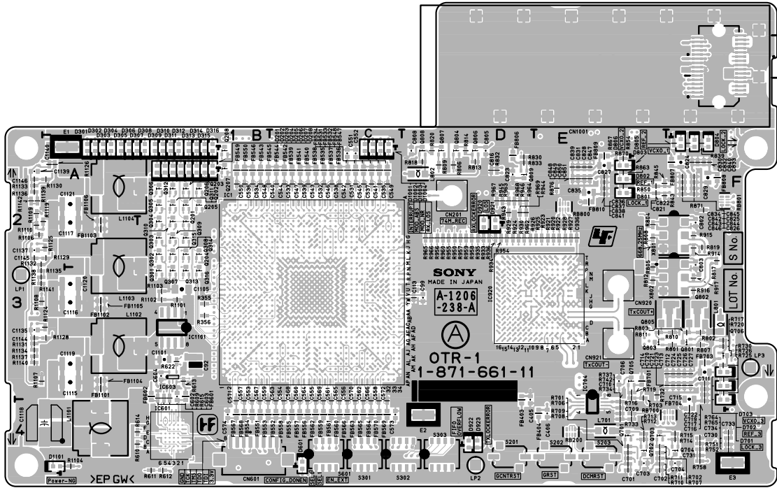
OTR-1 -A SIDE- SUFFIX: -11
