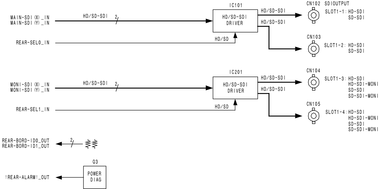
SDI OUTPUT HIF-25
