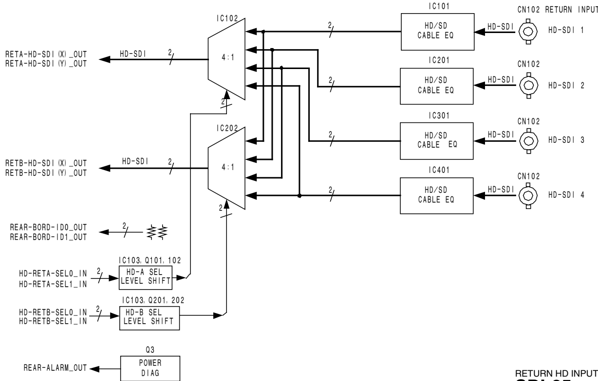
RETURN HD INPUT SDI-85
