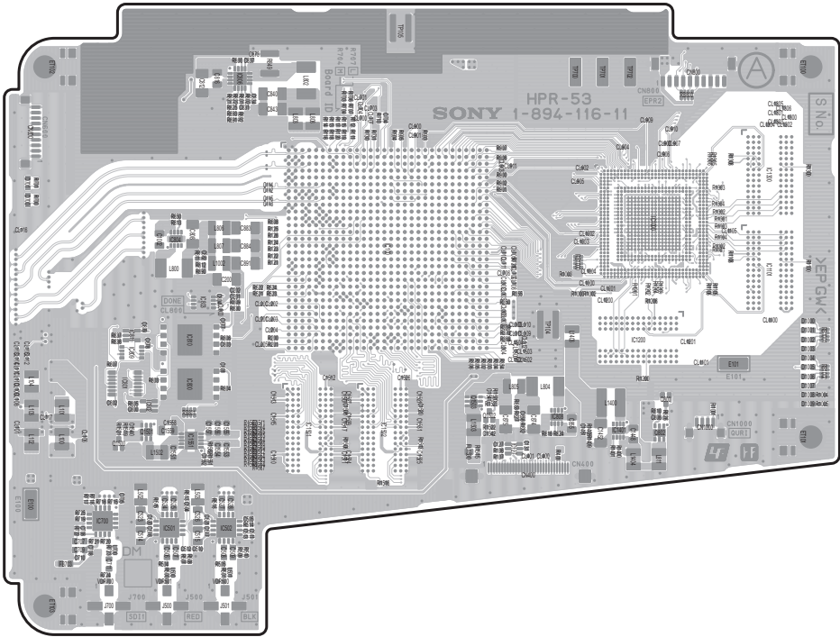
HPR-53 -A SIDE- SUFFIX: -11
