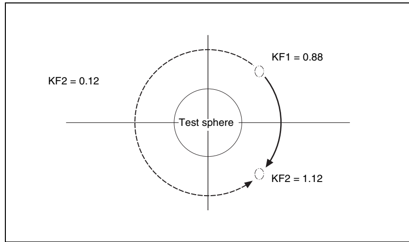
Keyframe trajectory
