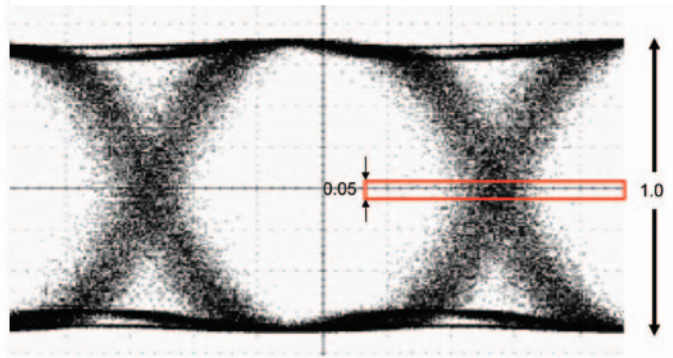
► Figure A-2. CSA803A histogram window.
