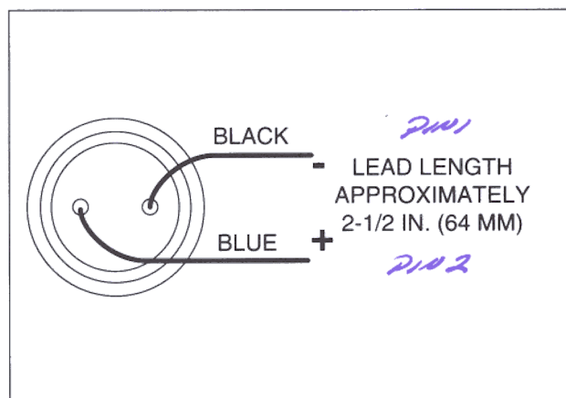
Wiring Diagrams
